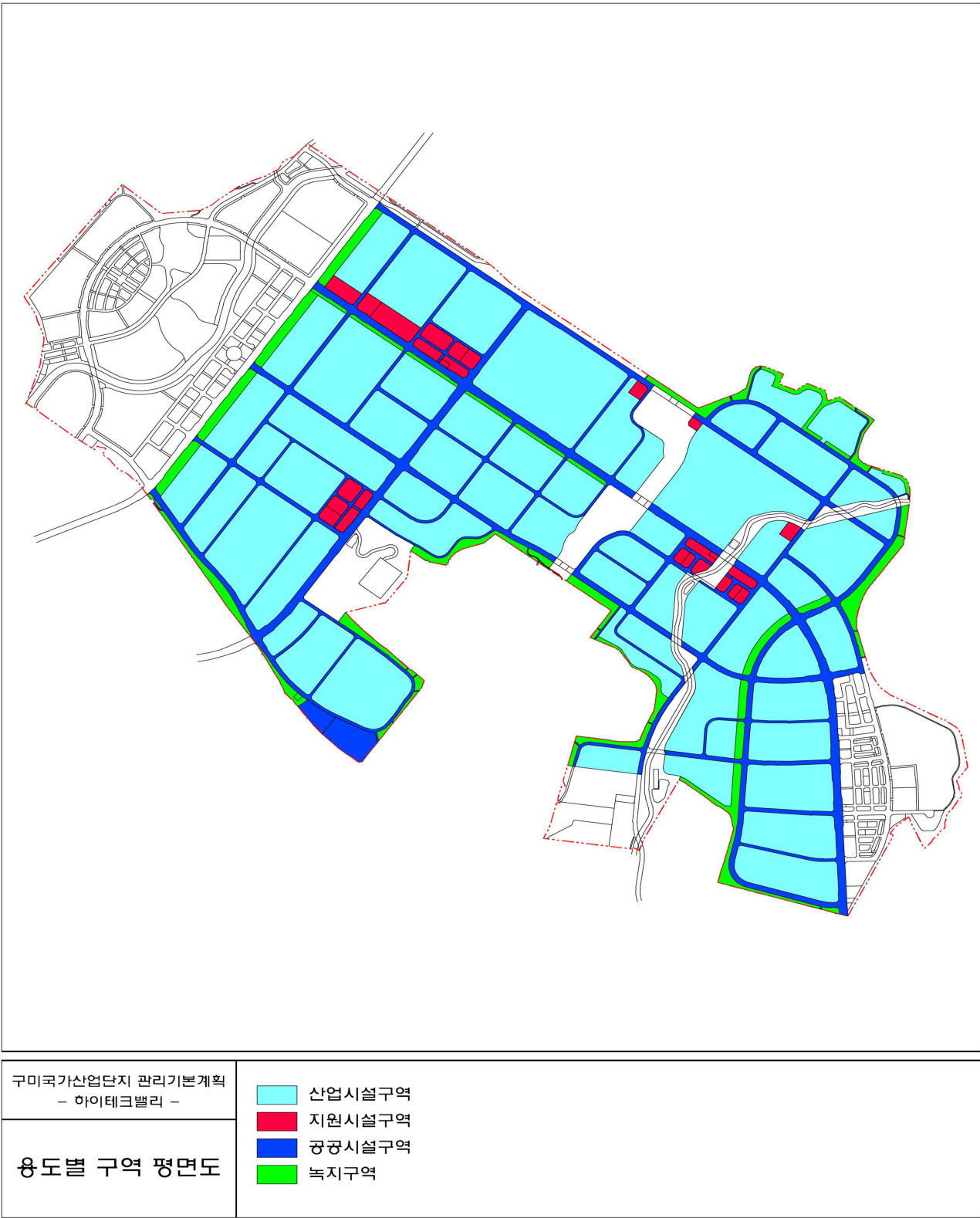
(별첨#2) 구미국가산업단지 용도별구역 평면도(하이테크밸리)
